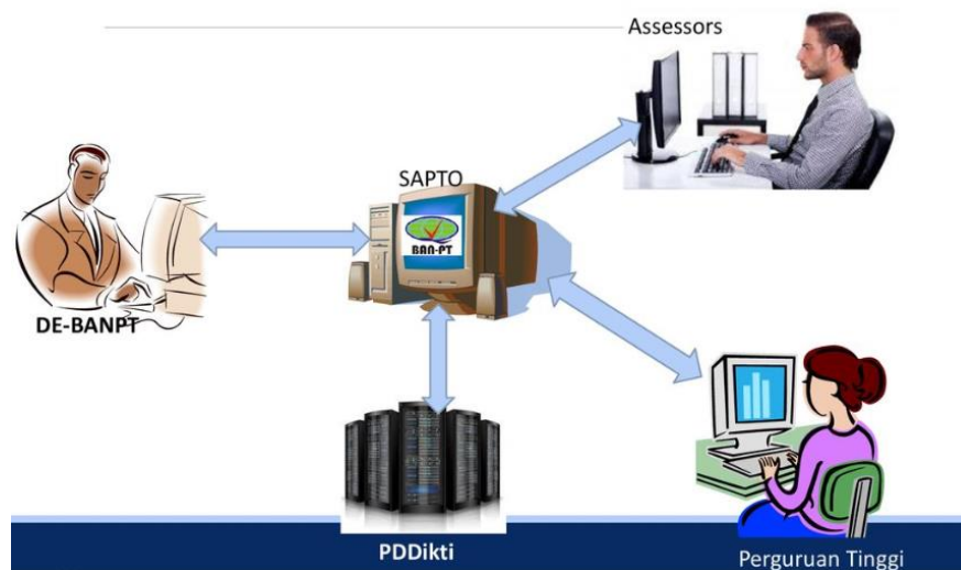
Gambar 8.4 Arsitektur SAPTO
